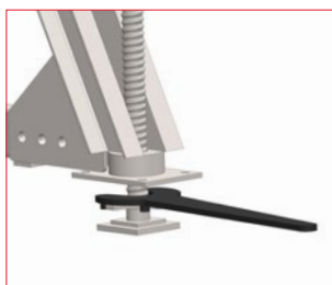
Ključ za podešavanje konzole jednostrane oplaste „S“
