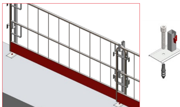
S nogom za zaštitnu ogradu i stupom za zaštitnu ogradu Pričvršćivanje sidrenim vijkom, tiplom 16 mm ili sidrenom čahurom i sidrenim vijkom DW15
