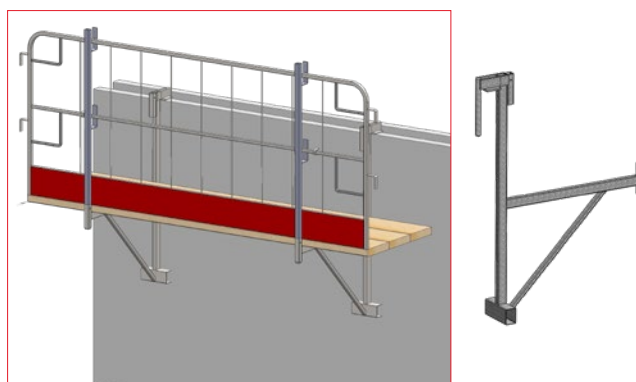
S univerzalnom spojnicom na parapetu Raspon podešavanja 50-450 mm
