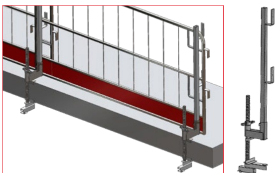
S univerzalnom spojnicom na rubu stropa Raspon podešavanja 50-450 mm
