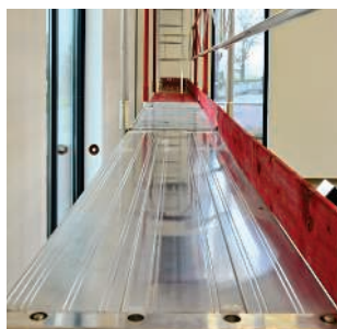
Celohliníkové podlahy 2,50 x 0,60 m 450 kg/m 2 3,00 x 0,60 m 200 kg/m 2
