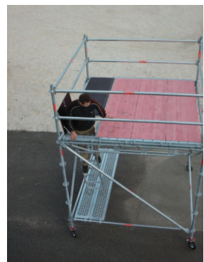
Pojízdná plošina
