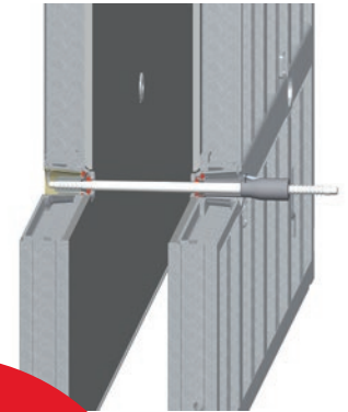
Master PRO detalj ankera
