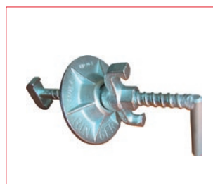
RS spojka
