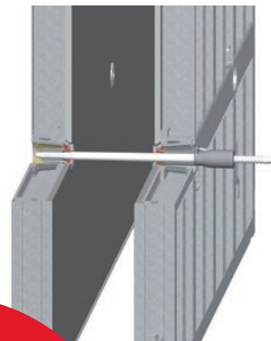
Detalj vezave Master PRO
