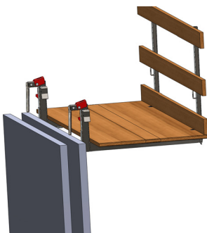
Bei Fertigteilwänden
